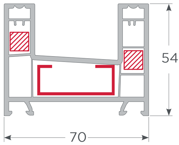
con Apoyo cerradero 9x9 - M Marco Doble Riel Corredera
