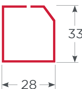
Ref. Box Marco Fijo Inclinado S60 1.2mm - TC PL-S60-TC-BMF-12
