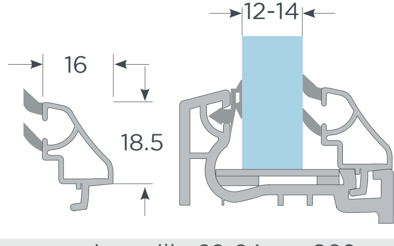
con junquillo 22-24mm S60 Acristalamiento 12-14mm
