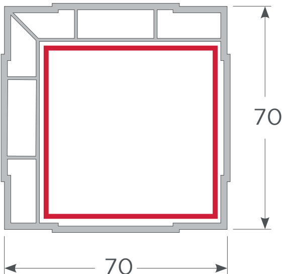
Esquinero 90° - 70mm Corredera
