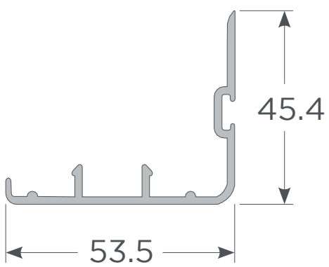
con Apoyo cerradero 9x9 - M Marco Triple Riel Corredera
