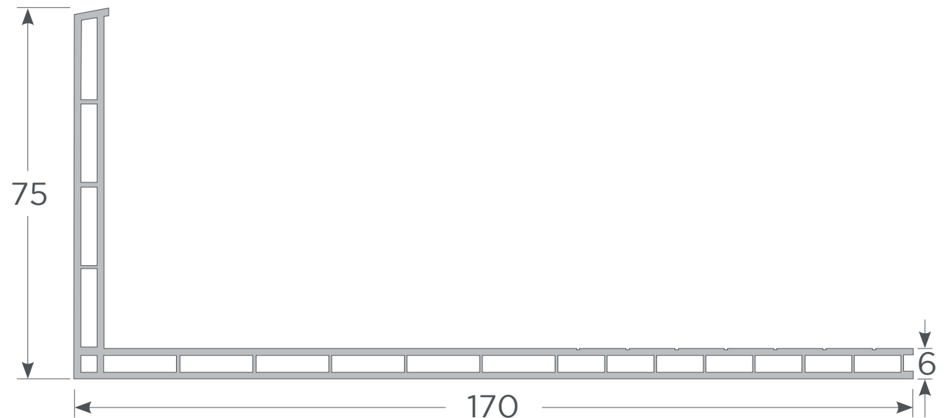
Ángulo de revestimiento 75 / 170mm
