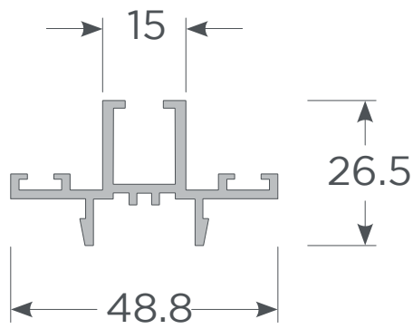
Adaptador Cuarta Hoja con Felpa
