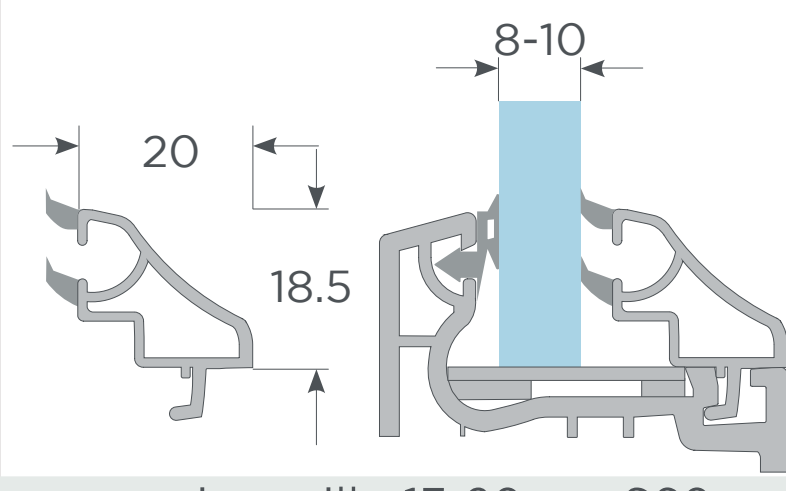
con junquillo 17-20mm S60 Acristalamiento 8-10mm
