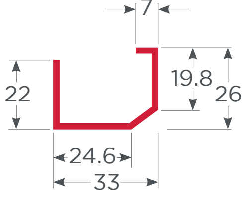
Ref. New Múltiple 2mm - TC PL-CMP-TC-MLT-2
